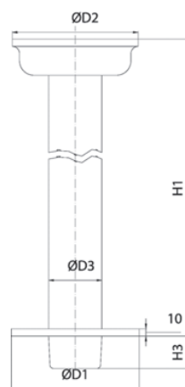
Стойка в сборе
